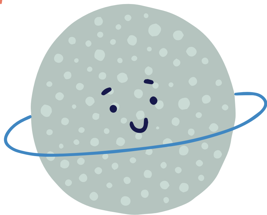
URANUS
