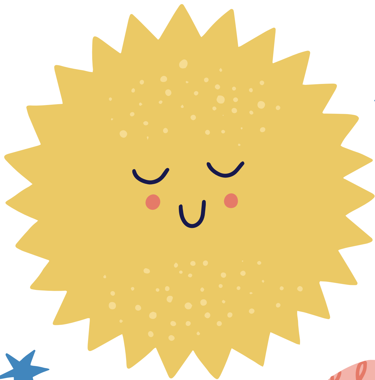
SUN
