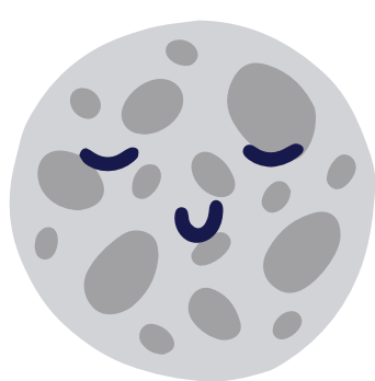
MOON
